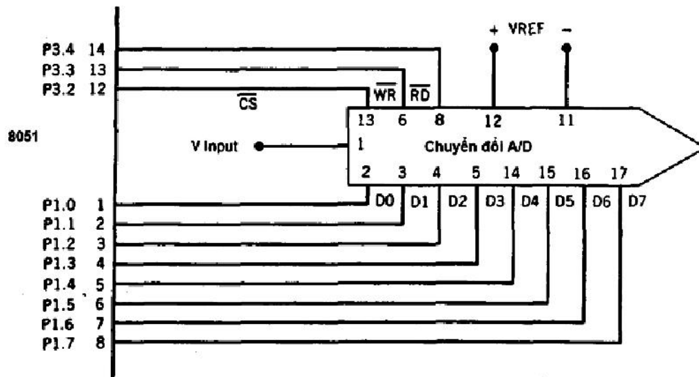
Hình 6-4. Gép nối 8051 và chuyển đổi A/D
