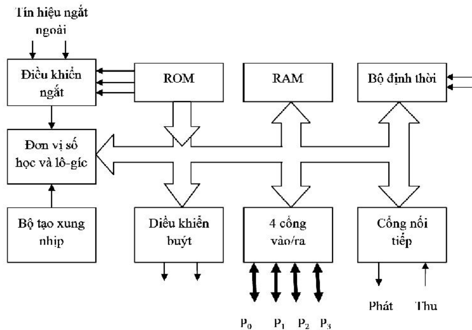
Hình 6-1. Sơ đồ khối 8051
