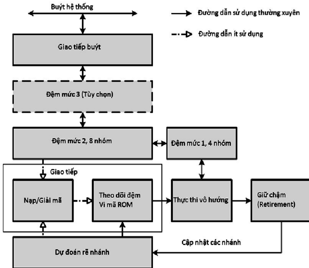
Hình 7-1. Vi kiến trúc Netburst
