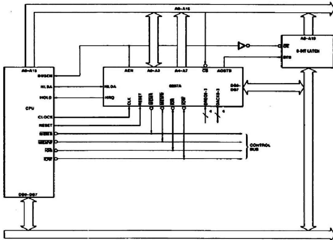
Hình 5-17. Ghép nối 8237 với bus hệ vi xử lý
