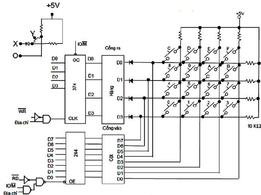
Hình 4-17. Ghép nối với bàn phím
