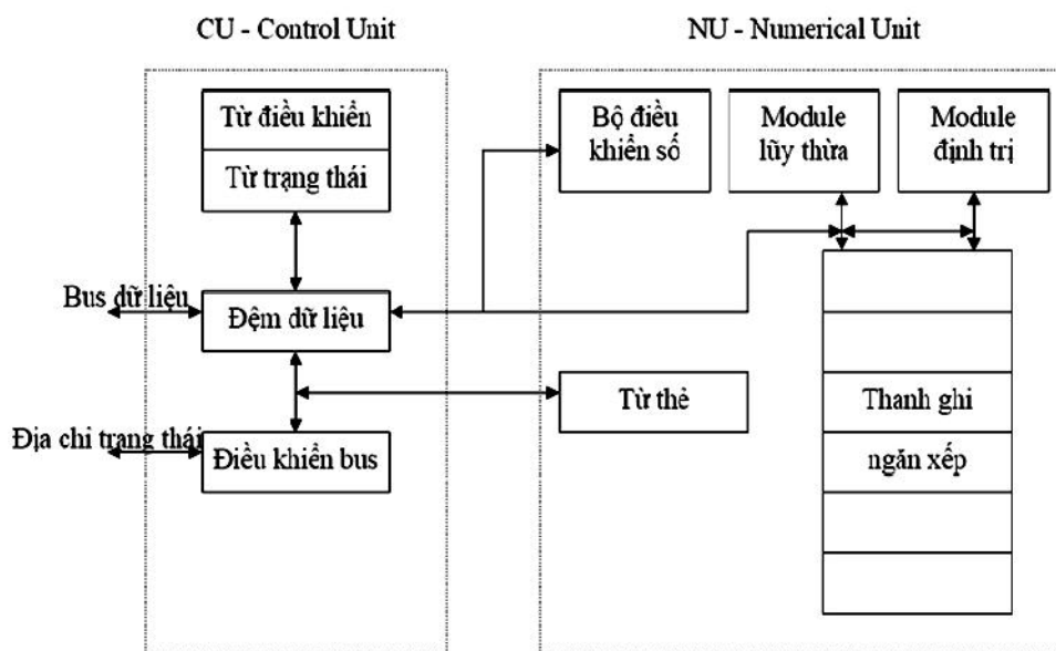
Hình 2-3. Sơ đồ khối 8087
