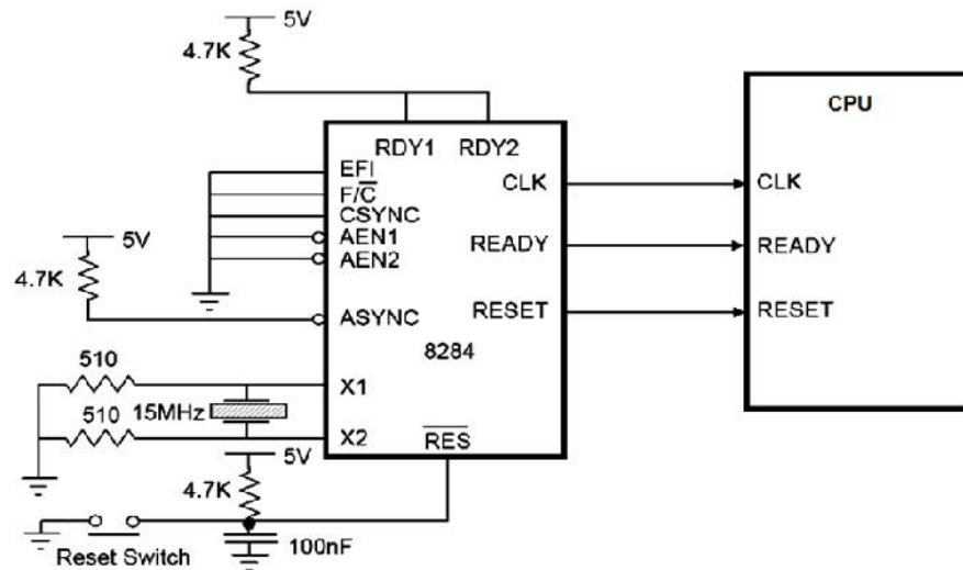
Hình 4-4. Ghép nối 8284 với vi xử lý
