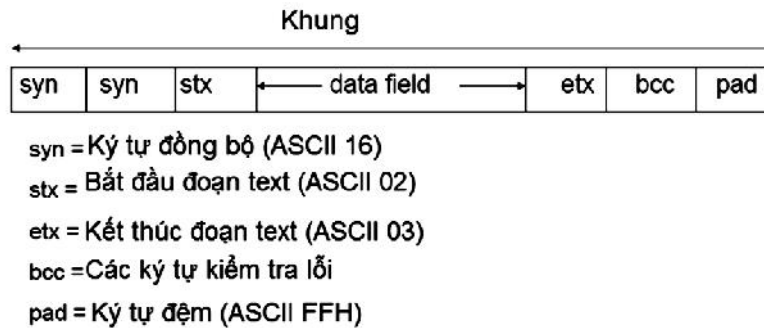
Hình 4-27. Cấu trúc khung đồng bộ
