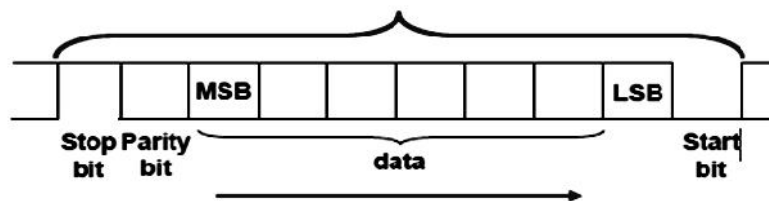
Hình 4-28. Cấu trúc dữ liệu truyền dị bộ
