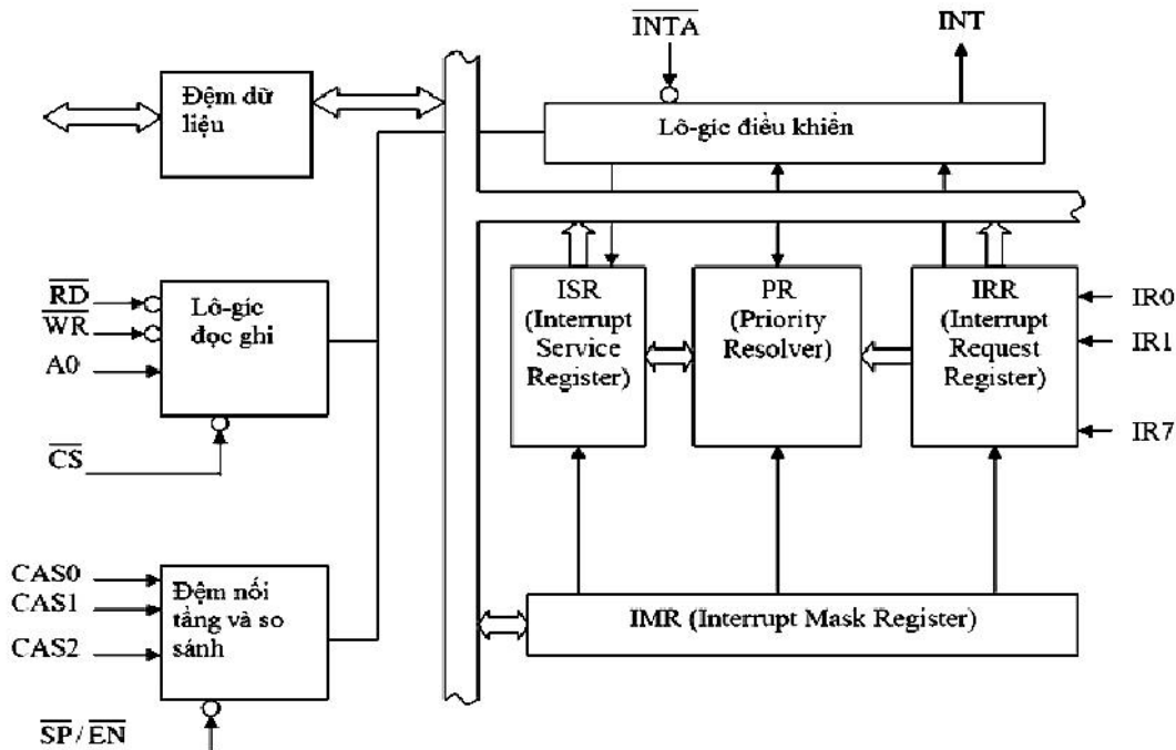
Hình 5-2. Sơ đồ khối 8259A
