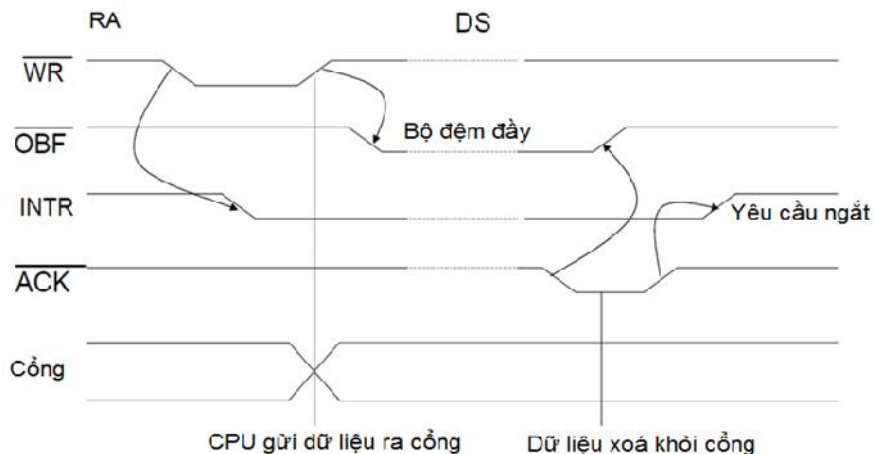
Hình 4-22. Biểu đồ thời gian tín hiệu ra
