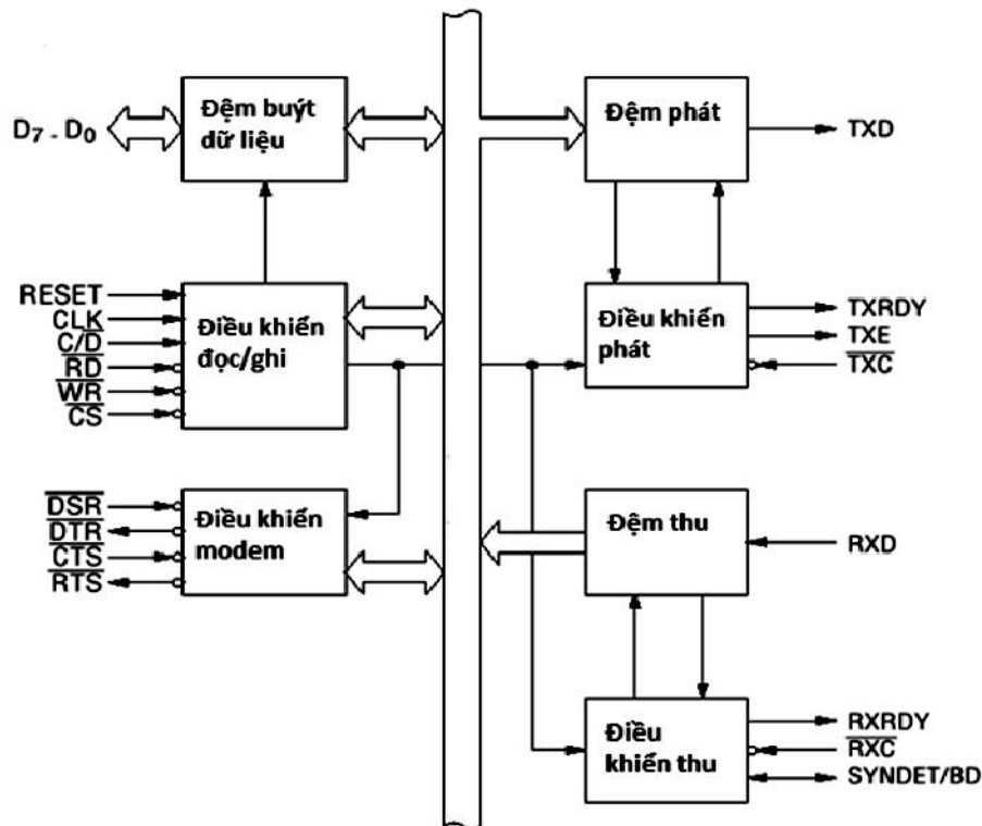
Hình 4-29. Sơ đồ khối 8251A
