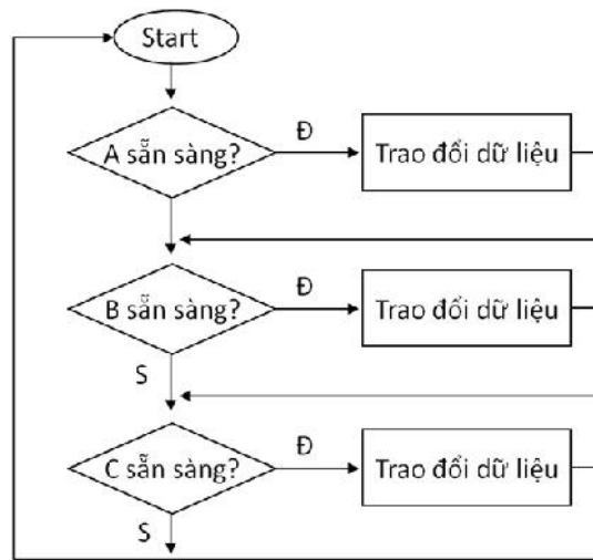
Hình 5-1. Vào/ra bằng thăm dò với nhiều thiết bị
