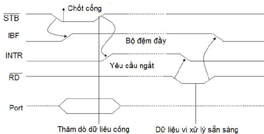
Hình 4-23. Biểu đồ thời gian tín hiệu vào
