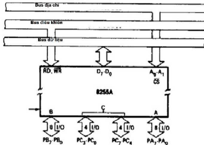
Hình 4-20. Các chế độ 0
