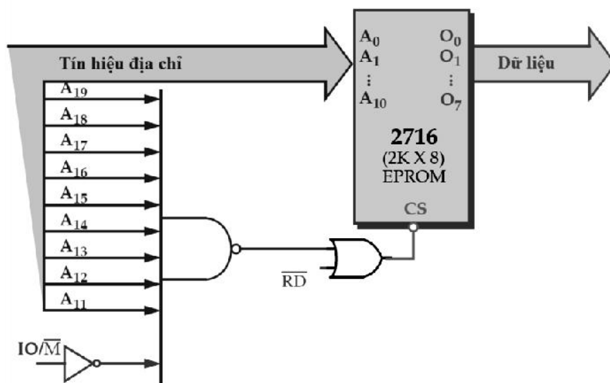
Hình 4-10. Mạch giải mã dùng mạch lô-gíc
