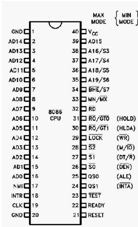
Hình 4-1. Các tín hiệu của 8086
