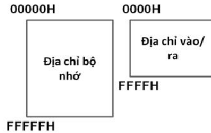
Hình 4-14. Không gian nhớ của thiết bị vào/ra và bộ nhớ chính
