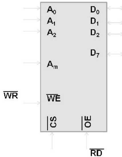
Hình 4-8. Vi mạch nhớ khái quát
