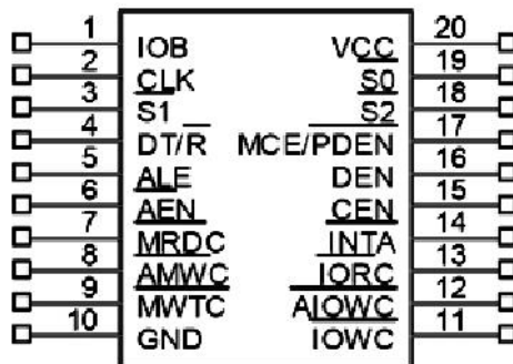
Hình 4-5. Bộ điều khiển bus 8288
