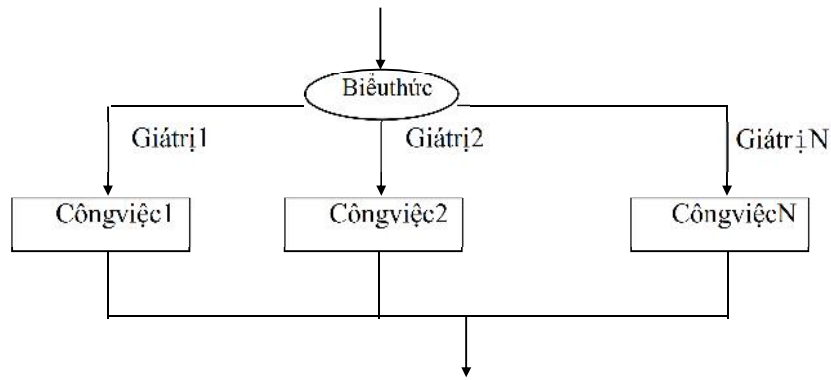
Hình 3-7. Cấu trúc lệnh CASE
