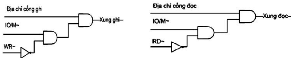
Hình 4-15. Giải mã thiết bị dùng cổng lô-gíc
