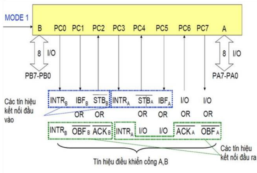
Hình 4-21. Ghép nối các tín hiệu điều khiển ở chế độ 1
