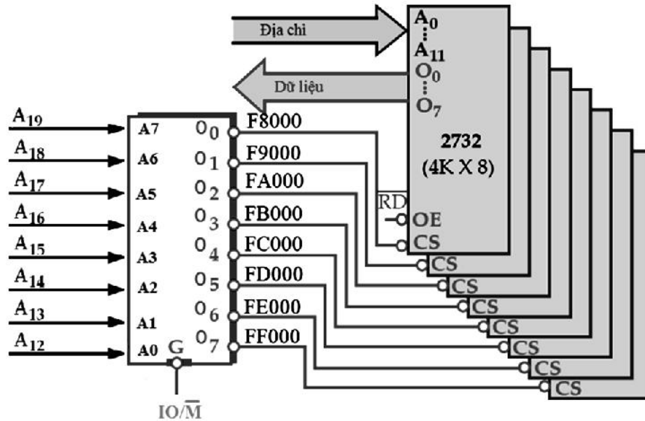
Hình 4-13. Giải mã dùng ROM
