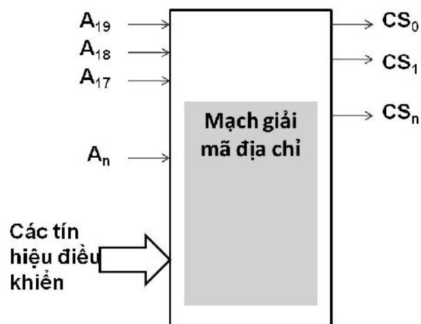
Hình 4-9. Mạch giải mã địa chỉ tổng quát
