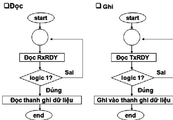
Hình 4-34. Lưu đồ đọc/ghi đơn giản
