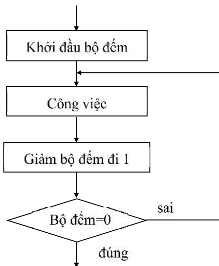
Hình 3-8. Cấu trúc lặp FOR - DO.
