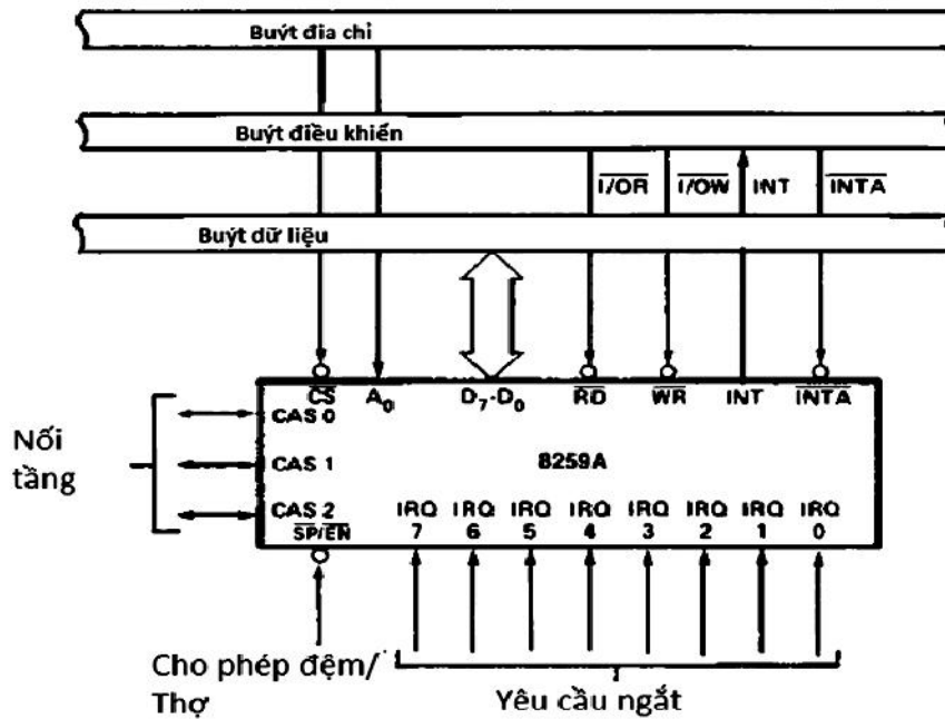
Hình 5-3. Ghép nối 8259 với bus 8086/8088
