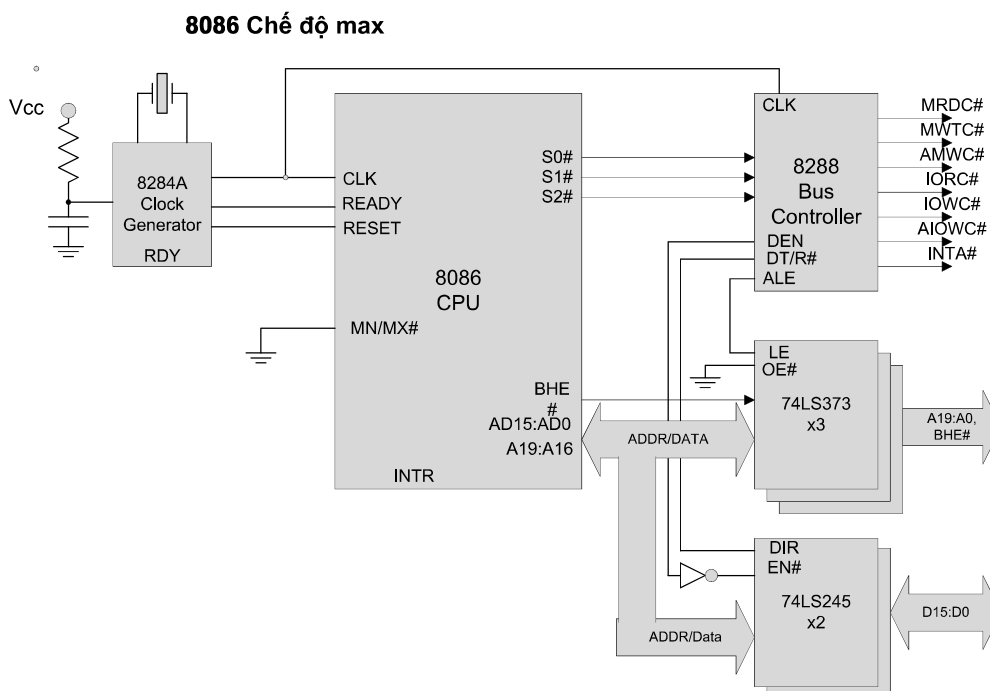
Hình 4-3. Bus hệ thống 8086 có đệm
