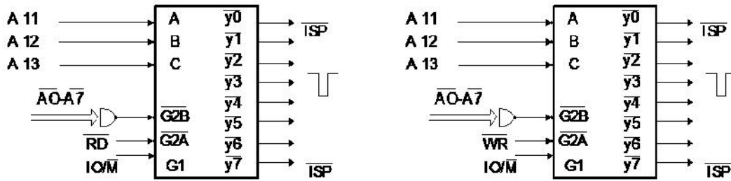
Hình 4-16. Giải mã địa chỉ cổng dùng 74LS138
