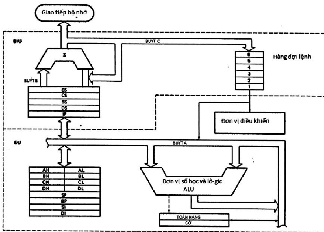
Hình 2-1. Sơ đồ khối 8086
