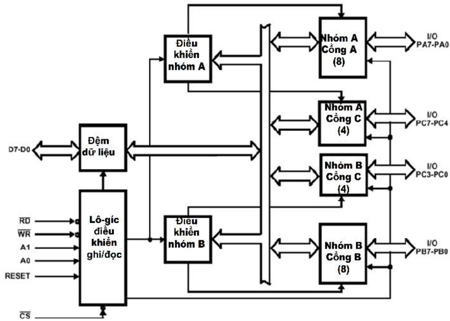
Hình 4-19. Sơ đồ khối 8255A
