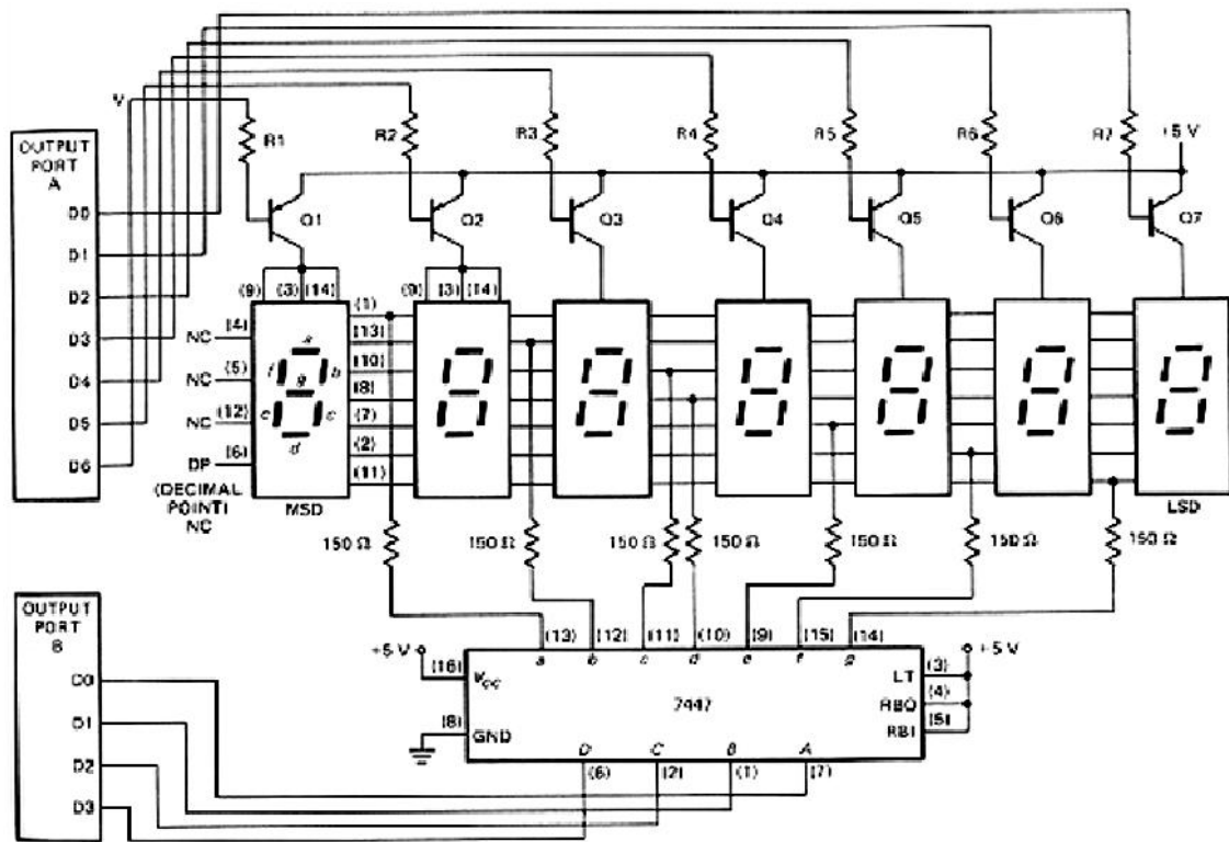
Hình 4-18. Ghép nối hiển thị số
